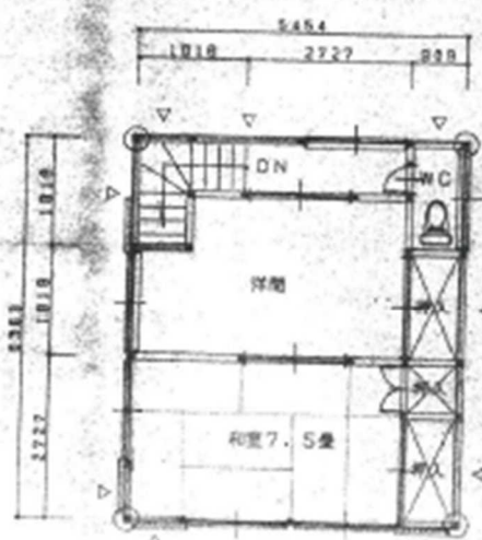
图 2-2 2 階平面図 縮尺 1/100
